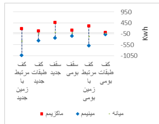
شکل ۱۲- بازه تغییر تبادل حرارتی سالانه سطوح افقی Figure 12- The range of annual energy exchange from horizontal surfaces
