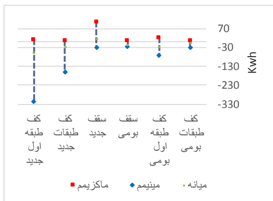
شکل ۸- بازه تبادل انرژی حرارتی سالانه سطوح افقی Figure 8- the range of annual energy exchange from horizontal surfaces
