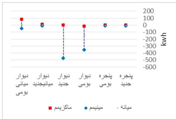
شکل ۱۲- بازه تبادل حرارتی سالانه سطوح عمودی Figure12- The range of annual energy exchange from vertical surfaces
