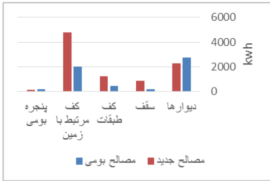
شکل ۱۱- مقایسه تبادل انرژی حرارتی سالانه سطوح مختلف Figure11- Comparison between the amount of thermal energy exchange
