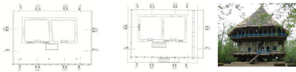
شکل ۴- تصویر و پلان خانه رفیعی (۱۹) Figure4- Image and plan of Mohtasham Talab house(19)
