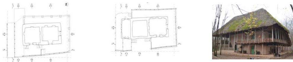
شکل ۱۴- تصویر و پلان طبقات خانه امینی (۱۹) Figure14- Image and plan of Amini house
