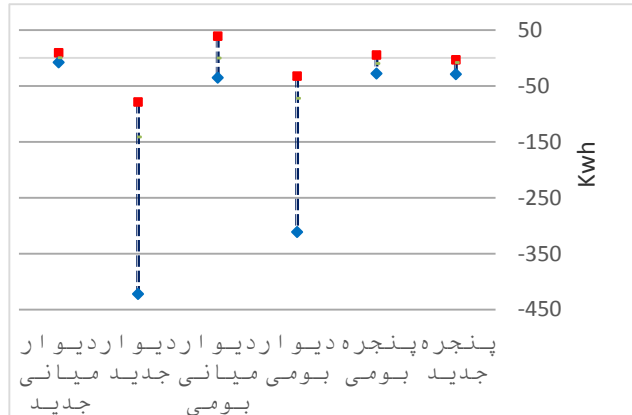
شکل ۷- بازه تبادل انرژی حرارتی سالانه سطوح عمودی Figure7- the range of annual energy exchange from vertical surfaces
