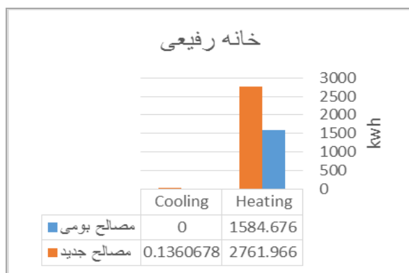
شکل ۵- مقایسه میزان مصرف انرژی گرمایش و سرمایش Figure5- Comparison between the amount of energy consumption for heating and cooling
