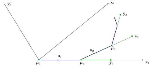
شکل ۲- روال هندسی الگوریتم LARS
