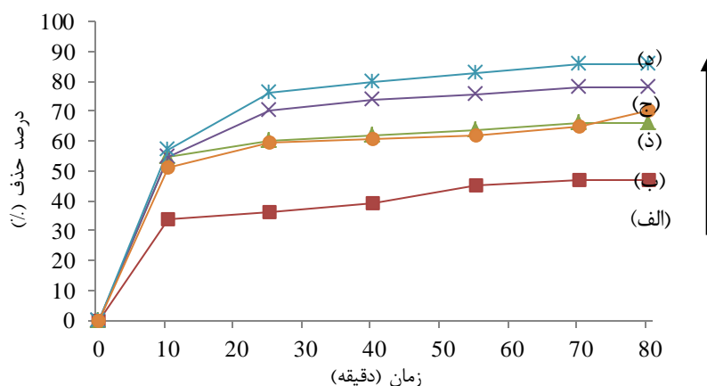
شکل ۴- فعالیت فتوکاتالیستی نانوذرات دی اکسید تیتانیوم (الف)، نانوکامپوزیت دی اکسید تیتانیوم / بنتونیت اولیه (ب) و دوپ شده با (ج) ۳، (د) ۵، (ه) ۱۰ درصد نقره در حضور نور فرابنفش.
