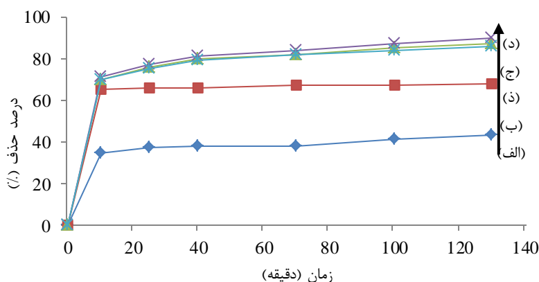
شکل ۵- فعالیت فتوکاتالیستی نانوذرات دی اکسید تیتانیوم (الف)، نانوکامپوزیت دی اکسید تیتانیوم / بنتونیت اولیه (ب) و دوپ شده با (ج) ۳، (د) ۵، (ه) ۱۰ درصد نقره در حضور نور مرئی.
