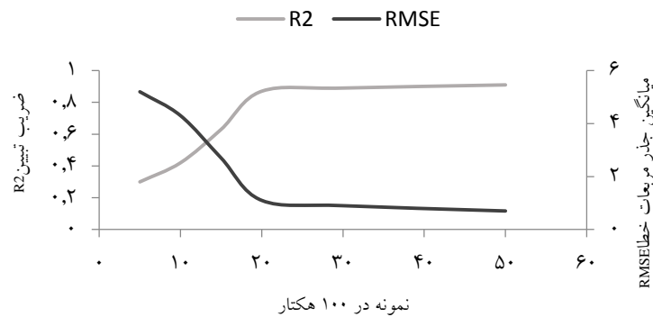
شکل ۳. نمودار تغییرات دقت تخمین برحسب تعداد حسگر استفاده شده
